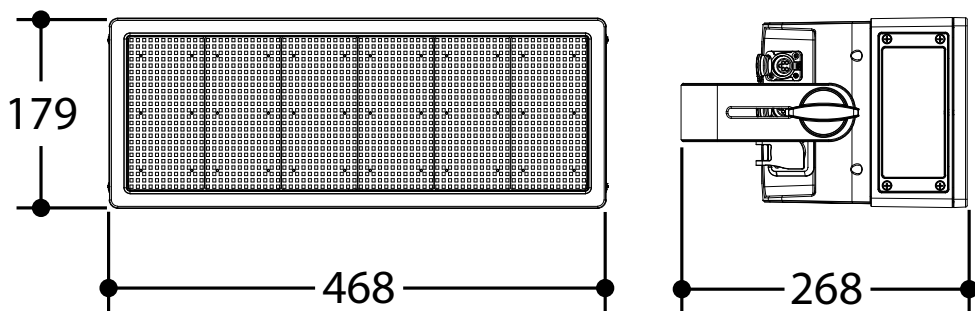
Disegno tecnico
